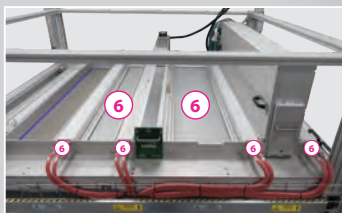
Widok z góry - Komora obojętna z regulowanymi wtryskiwaczami azotu
